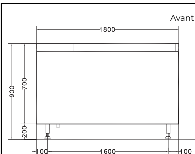
Côté
